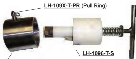
LH-109X-T-C (Steel Collar)
